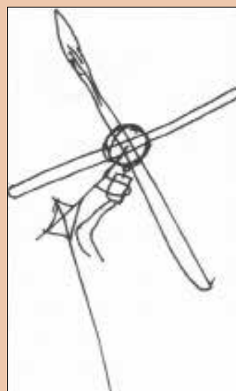
De eerste experimentele radiowindmolen die ik met Geoffrey maakte. Het succes van dit model gaf me de inspiratie om iets groters te maken. (Tekening William Kamkwamba).
