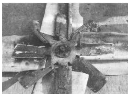
De trekkerventilator en wieken van mijn eerste grote windmolen. Deze foto is gemaakt nadat ik de Carlsberg-doppen door echte afsluitringen had vervangen en een paar nagels had toegevoegd, maar verder is alles hetzelfde. (Tom Rielly)
