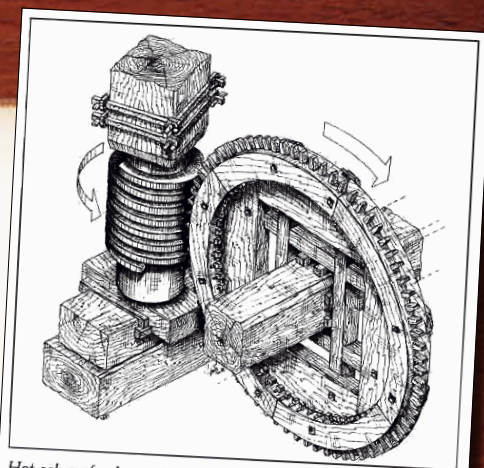
Het schroefrad van Jan Blauken, zoals het er waarschijnlijk zou hebben uitgezien, als het ooit zou zijn uitgevoerd. Het bezwaar ervan is, dat in de getekende uitvoering de koningsspij 23 omwentelingen moet maken tegen 1 omwenteling van het rad. Tekening Gerrit Pouw
