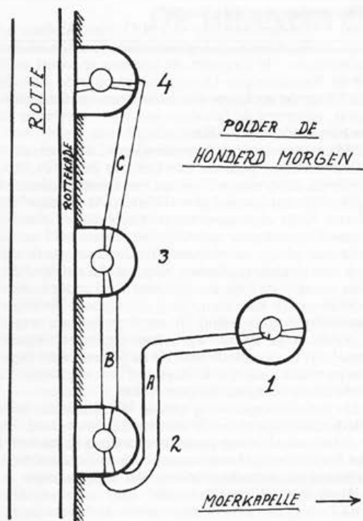
Afb. 3 Moerkapelle. Schema van de in 1925 gesloopte viergang schepradmolens. Molen 1 en 4 normaal. molen 2 en 3 malen 'links'.
