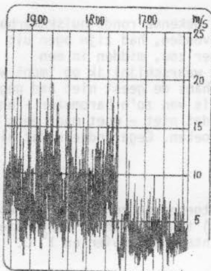
Figuur 3. Windregistratie te Amersfoort 1.11.1986
